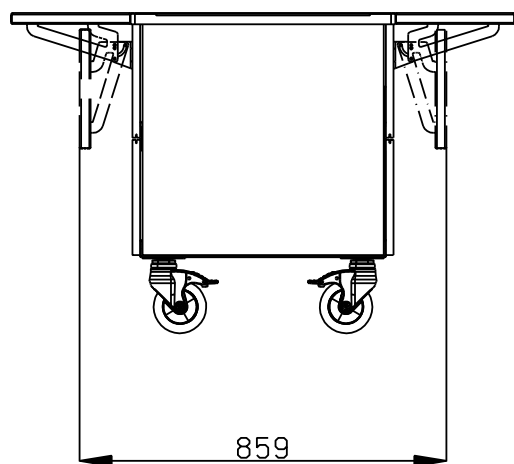
Bočna/o
